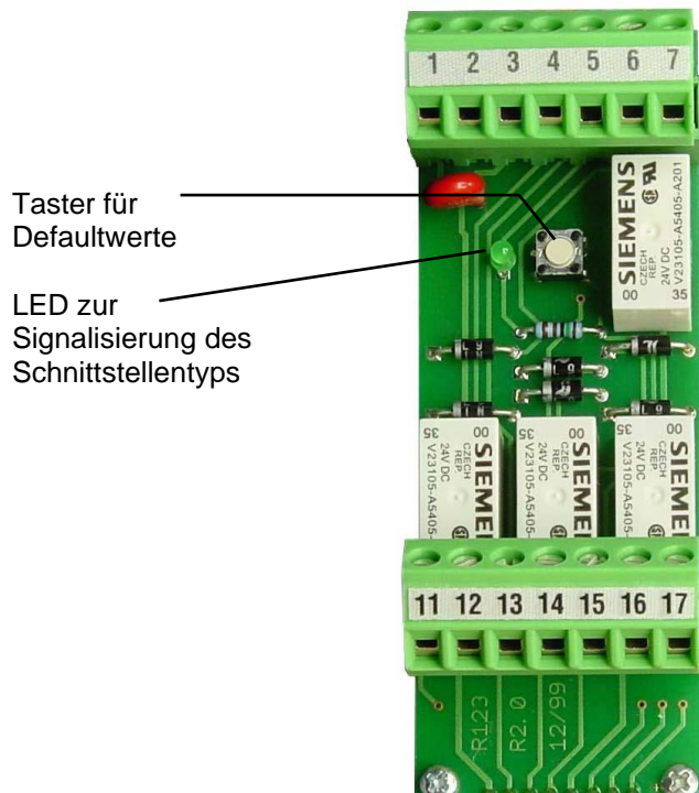
Abb. 4.5: LED zur Anzeige des konfigurierten Schnittstellentyps und Taster zum Einstellen der Defaultwerte
