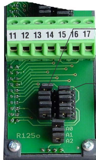
Abb. 5.1: Jumper zur Codierung von Arbeits- und Ruhestrom sowie LED-Farbe Rot/Grün auf SBLM1001
