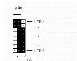
Abb. 4: Jumper Position für die LED-Farbe LED 1..8 am JDB1620 (LEDs 9..16 entsprechend)
