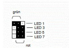
Abb. 4: Jumper-Position für die LED-Farbe am JDB8420
