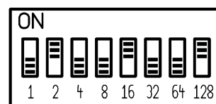
Abb. 2: Einstellen der Bus-Adresse
