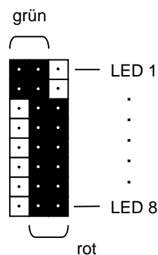
Abb. 4: Jumper-Positionen für LED-Farben an JDB8020 und JDB8040
