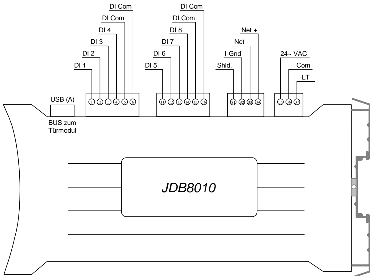
Abb. 1: Anschlussplan des Moduls JDB8010
